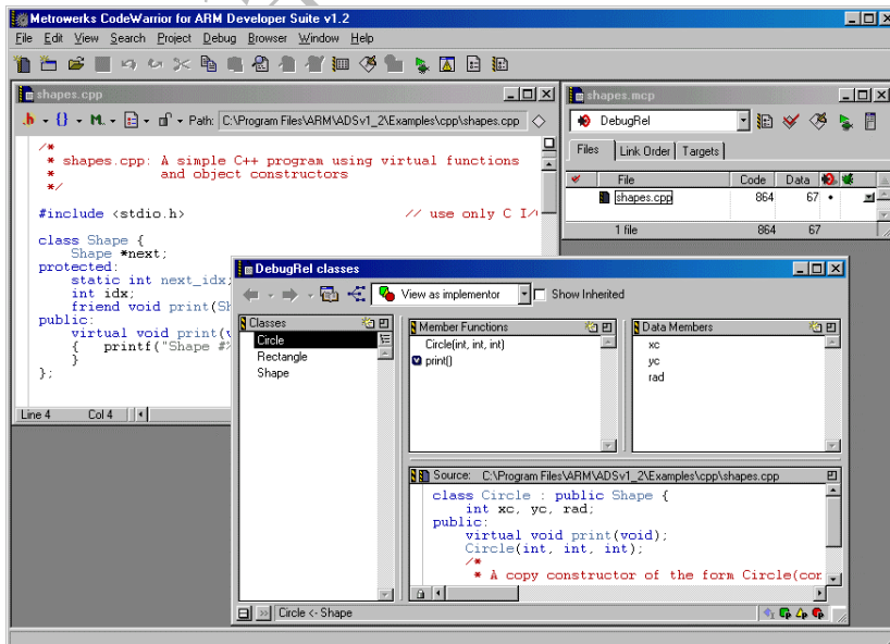
图 1.2 CodeWarrior 集成开发环境
