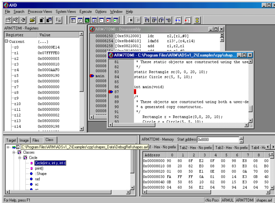
图 1.3 AXD 图形界面
