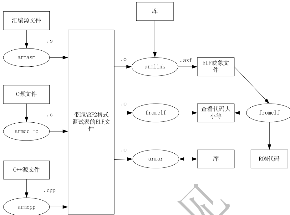
图 1.1 ARM 开发工具组件使用过程
