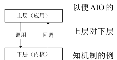
图 9.3 回调与调用
